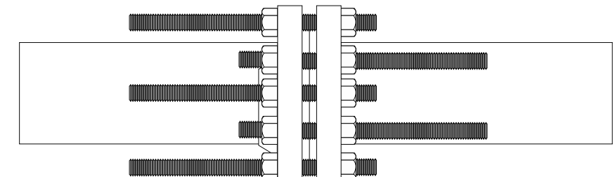
Configuración de tensionado al 100% para tensionado submarino
