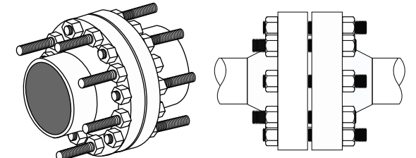
Tensionado de un 100% de los pernos
